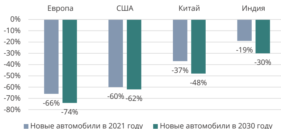
Рисунок-3. Предполагаемое сокращение выбросов ПГ в течение жизненного цикла новых электромобилей среднего размера по сравнению с автомобилями на бензине
